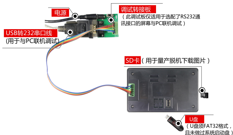
图 1-4 RS232 调试图
