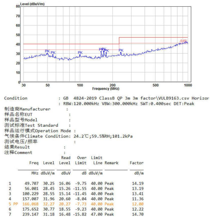
图 7-7 辐射测试垂直方向
