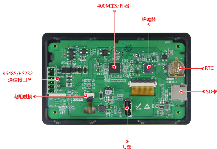
图 1-2 硬件配置图
