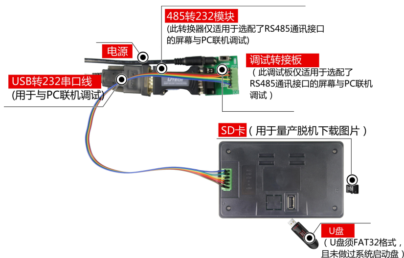
图 1-3 RS485 调试图
