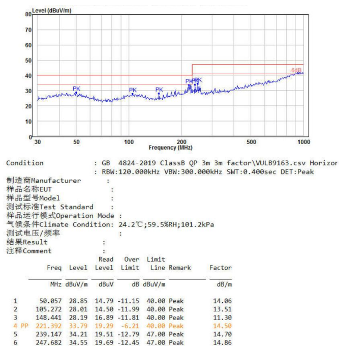
图 7-6 辐射测试水平方向
